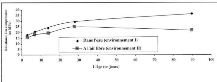
Figure 3 : Évolution de la résistance à la compression dans les deux milieux.
