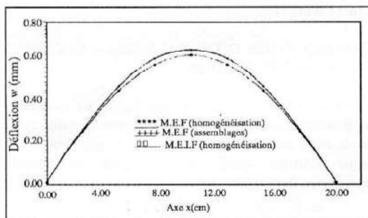
Figure 1 : Plaque carrée appuyée simplement courbes comparatives de la variation de la déflexion suivant l'axe x pour y = b/2 .
