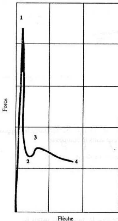
Figure 10 : Courbe force-flèche obtenue lors d'un essai de flexion.
