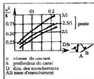
Courbe de dimensionnement des enrochements
