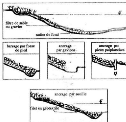
Figure 1 : Protection des berges et du lit par des matériaux minéraux
