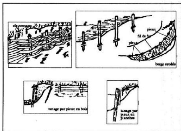
Figure 4 : Protection des berges par du matériel végétal.
