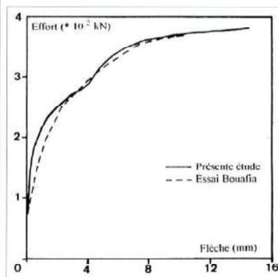
Figure 7: Evolution de la flèche au tiers de la travée en fonction de la charge P.
