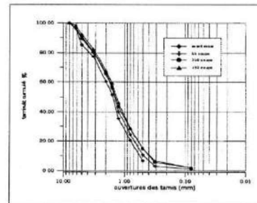
Figure 3 : Etalement des courbes granulométriques en fonction du nombre de coups pour la classe granulaire 0/6 à l'état humide.
