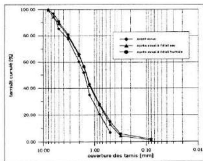
Figure 7 : courbes granulométriques de la classe granulaire 0/6 aux états sec lâche et humide pour 55 coups
