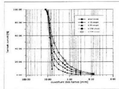
Figure 6 : évolution de la dégradation des grains en fonction du nombre de coups pour la granulométrie 6/10 à l'état humide
