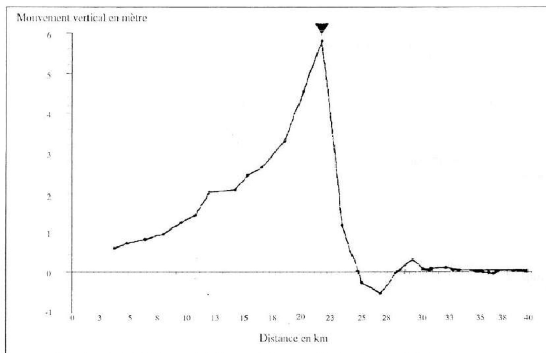
Figure 4 : Cheminement du nivellement général le long de la voie ferrée, Alger-Oran, traversant la faille générée par le séisme d'El-Asnam du 10 Octobre 1980.
