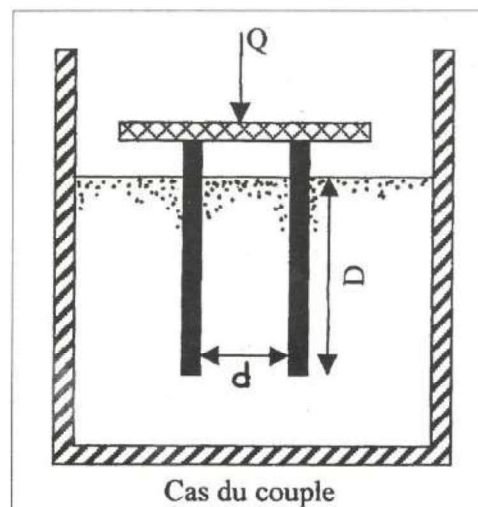
Figure 6 : Disposition schématique d'un couple de pieux
