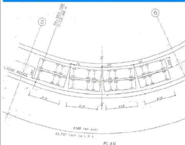
figure n° 1- Chargement de la travée centrale P5-P6
