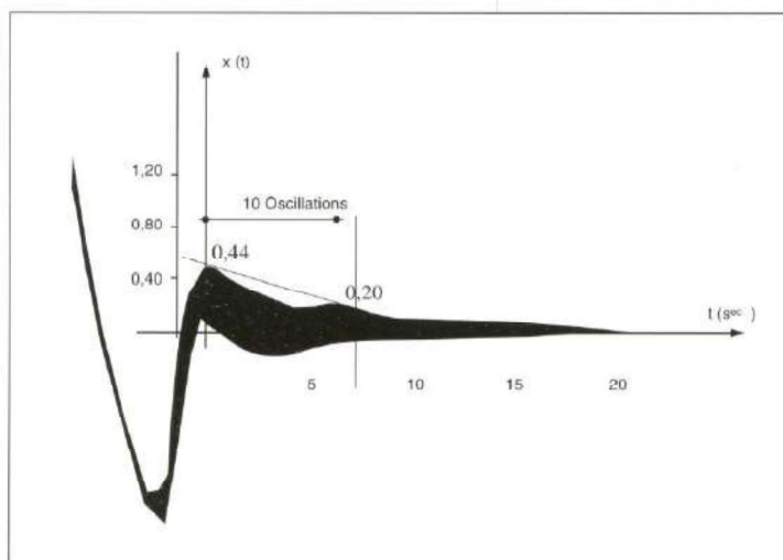
figure n°5- Amplification de la phase d'oscillation libre amortie
