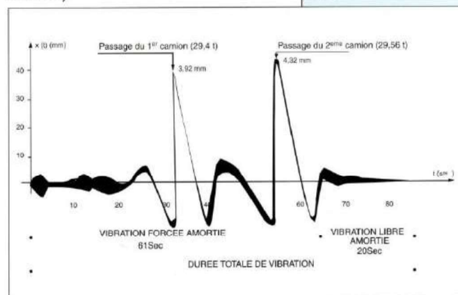
figure n°4- Amplification du spectre de réponse de la travée P5-P6
