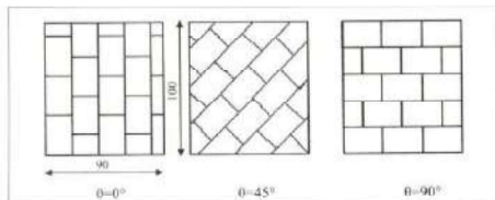
Figure 1 : Dimensions des murets en briques de terre cuite creuses
