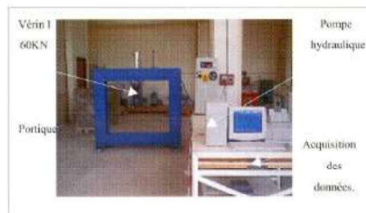
Photo 1 : Ensemble du dispositif d'essai
