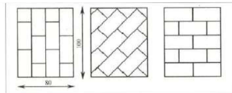
Figure 2 : Dimensions des murets en parpaings
