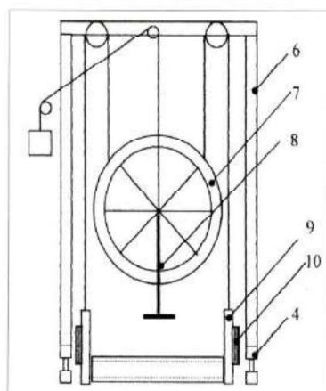
Figure 1 : Installation expérimentale
