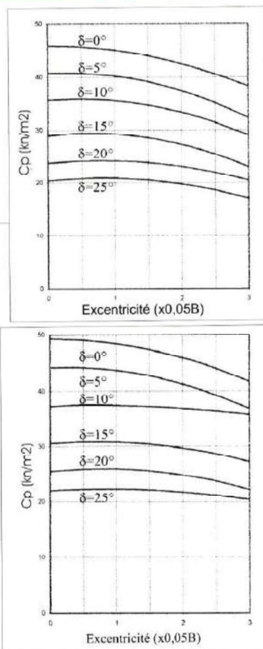
Figure 4 : Relation portance-excentricité (Fondation en caissons).
