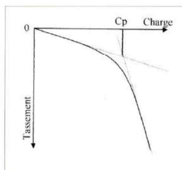
Figure 2 : Schéma de détermination de la capacité portante d'un sol.
