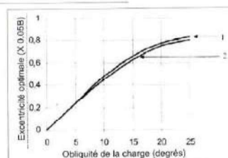
Figure 5 : Relation portance optimale-obliquité 1- Fondation en caissons; 2- Fondation rectangulaire.
