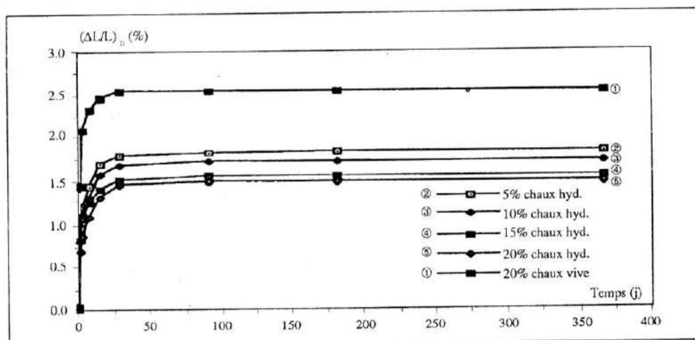
Figure 1 : Retraits de constitution (\Delta L/L_0)_n = (L_0 - L_n)/L_0 en fonction du temps ( L_0 : longueur de l'éprouvette après extrusion, L_n : longueur à n jours de conservation en salle régulée).
