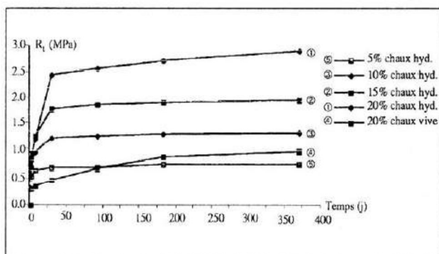
Figure 3 : Résistances à la traction par flexion R_x en fonction du temps.
