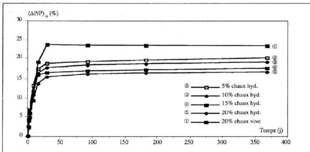
Figure 2 : Pertes de poids de constitution (\Delta P/P)_n = (P_0 - P_n)/P_0 en fonction du temps ( P_0 : poids de l'éprouvette après extrusion, P_n : poids à n jours de conservation en salle régulée).
