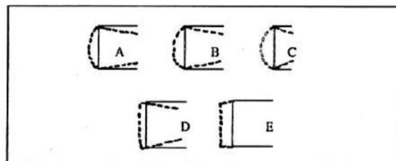
Figure 4 : Modes d'instabilité du profil U1.
