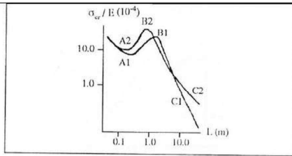
Figure 12 : Contraintes critiques en fonction de la longueur de la demi-onde du profil U5 (modes symétrique et antisymétrique).
