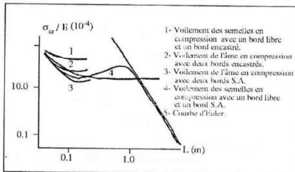
Figure 14 : Comparaison des résultats théoriques avec ceux de la méthode des bandes fines.
