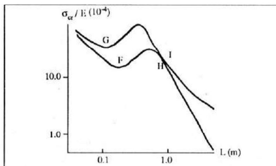
Figure 5a : Contraintes critiques en fonction de la longueur de la demi-onde du profil U1 (modes symétrique et antisymétrique).
