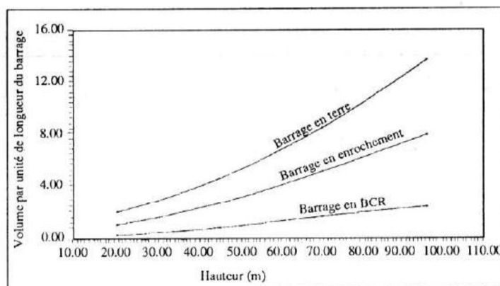
Figure 3 : Evolution des besoins en matériau.
