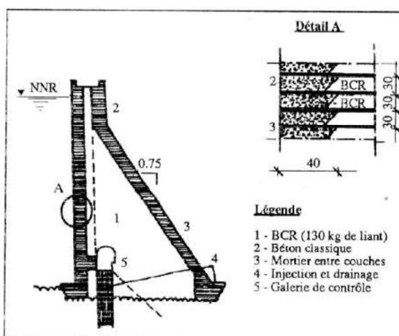
Figure 1 : Barrage en BCR. Section type.
