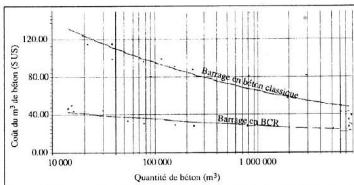
Figure 2 : Evolution du coût du m 3 de béton.
