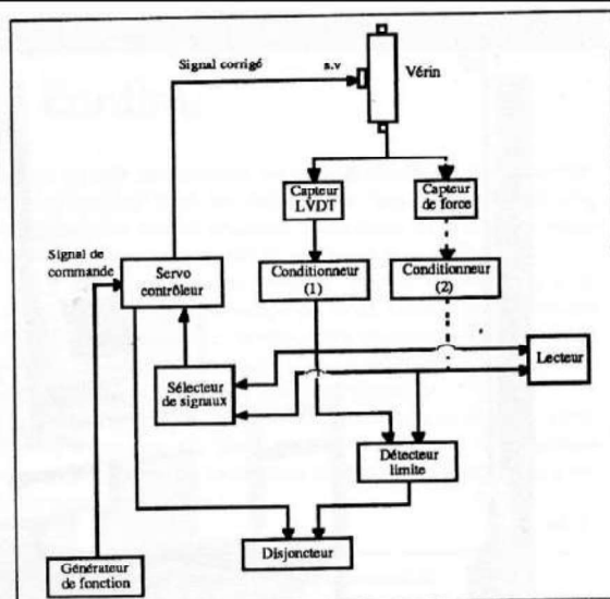
Figure 3 : Diagramme de l'unité de contrôle de base.
