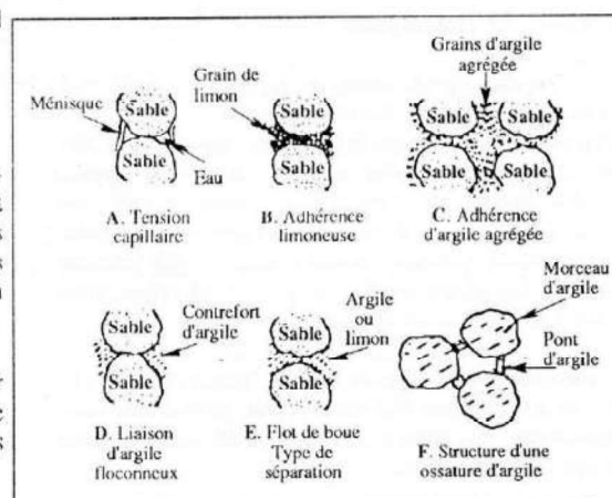
Figure 1 : Structures typiques de sol susceptible d'affaissement (Clemence et Finbarr, 1981).
