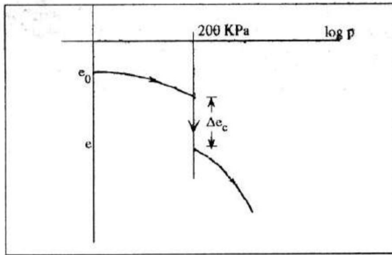
Figure 2 : Résultat de test du potentiel d'affaissement typique (Clemence et Finbarr, 1981).
